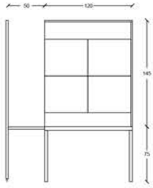
Ön Görünüş 1/50
