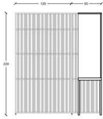
Yan Görünüş 1/50
